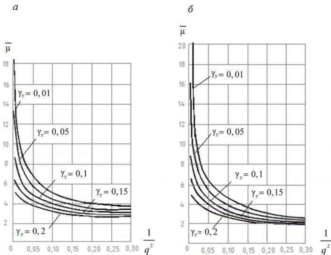
a – остановочный режим; b – пусковой режим
